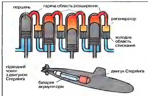
Двигун Стерлінґа Будова та застосування
